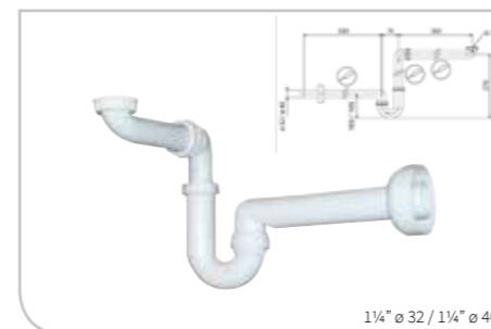
Raumsparsiphon Space-saving siphon
